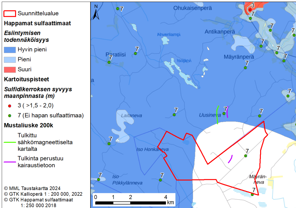
Kuva 13 Happamat sulfaattimaat.
