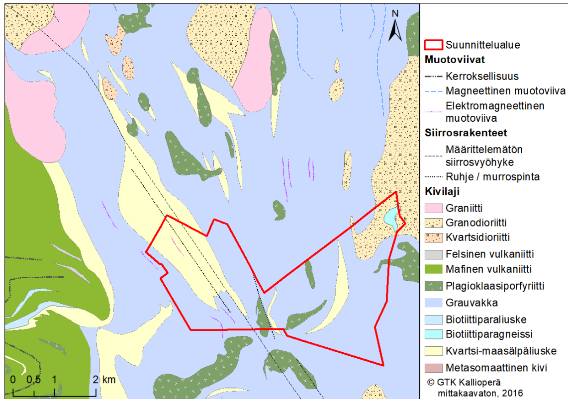
Kuva 11 Suunnittelualueen kallioperä.
