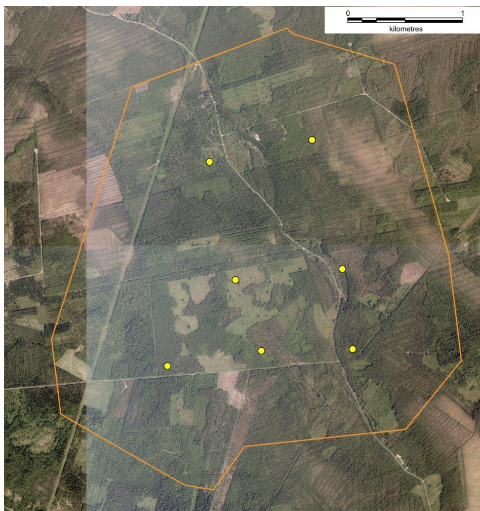
Kuva 2. Kesonmäen tuulivoimapuiston yleiskaava-alue ja voimalasijoittelu.
